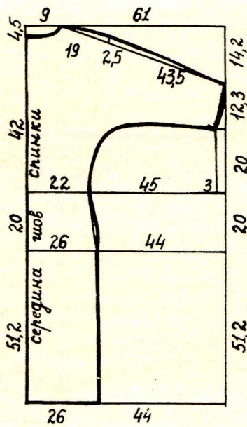
Спинка 2дет.
