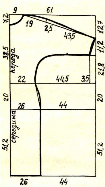
Деталь переда
